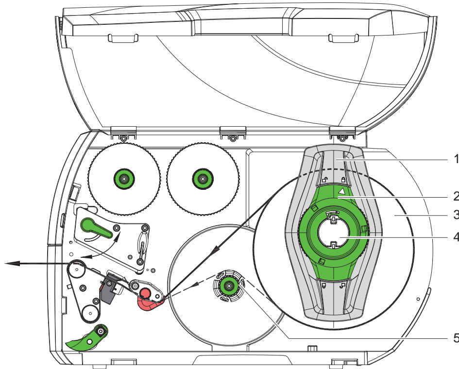
Figure 12 Insertion du rouleau d'étiquettes
