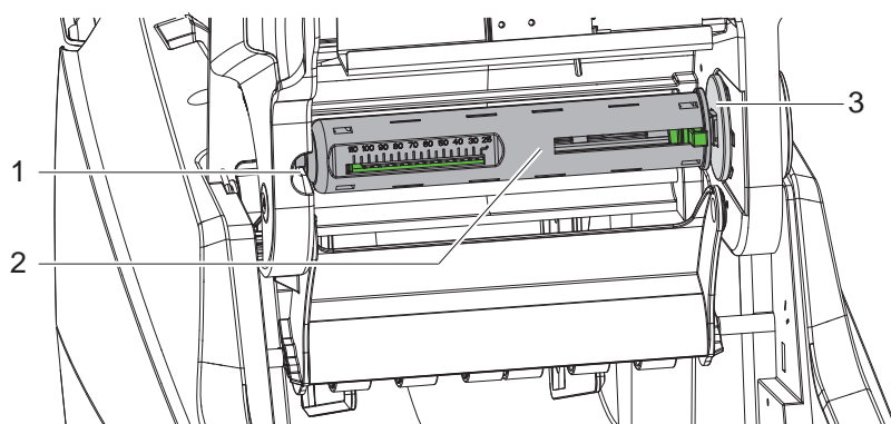
Figure 18 Retrait de l'axe du ruban transfert du dérouleur
