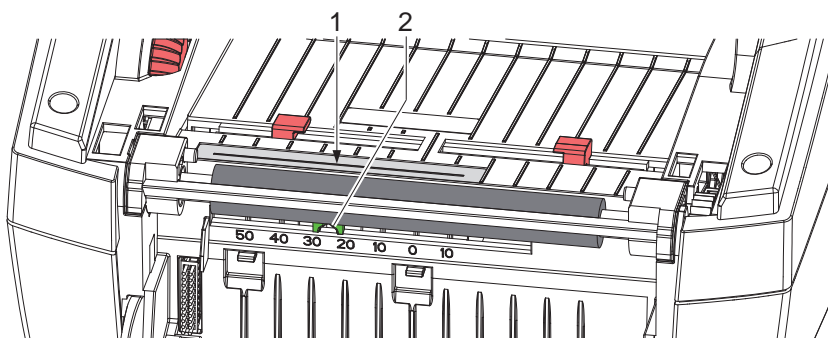
Figure 17 Positionnement de la cellule réflexe
