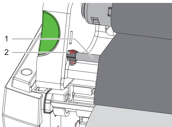
Figure 21 Réglage du défilement du ruban transfert
