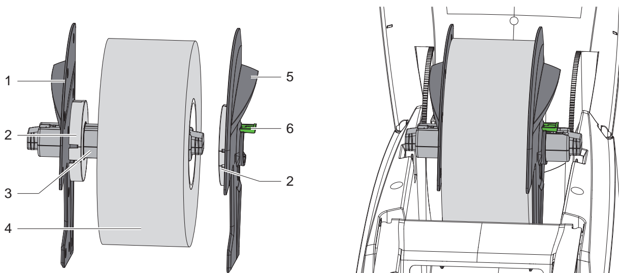
Figure 11 Insertion du rouleau d'étiquettes
