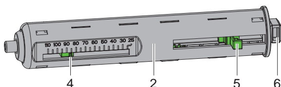
Figure 19 Ajustement de l'axe de ruban transfert
