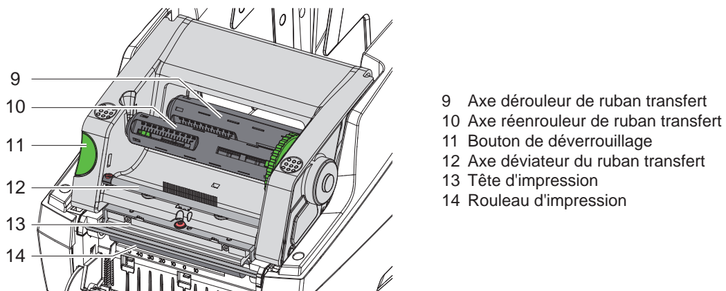
Figure 2 Mécanisme d'impression
